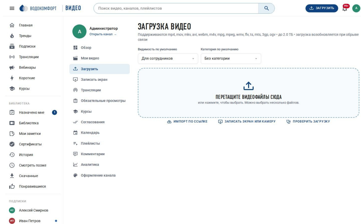
Рис. 32. Загрузка видео
