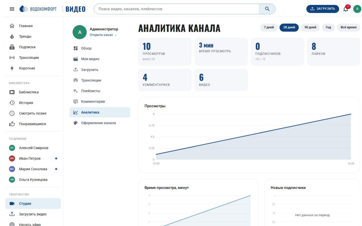
Рис. 35. Аналитика канала
