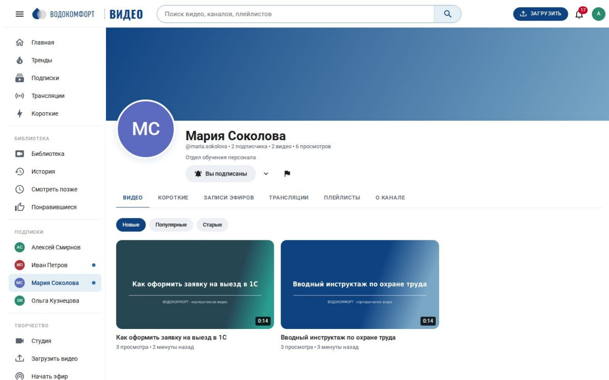
Рис. 36. Страница канала
