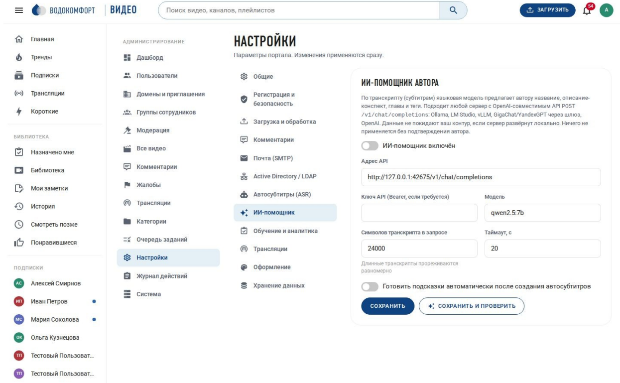
Рис. 55. Настройки → ИИ-помощник
