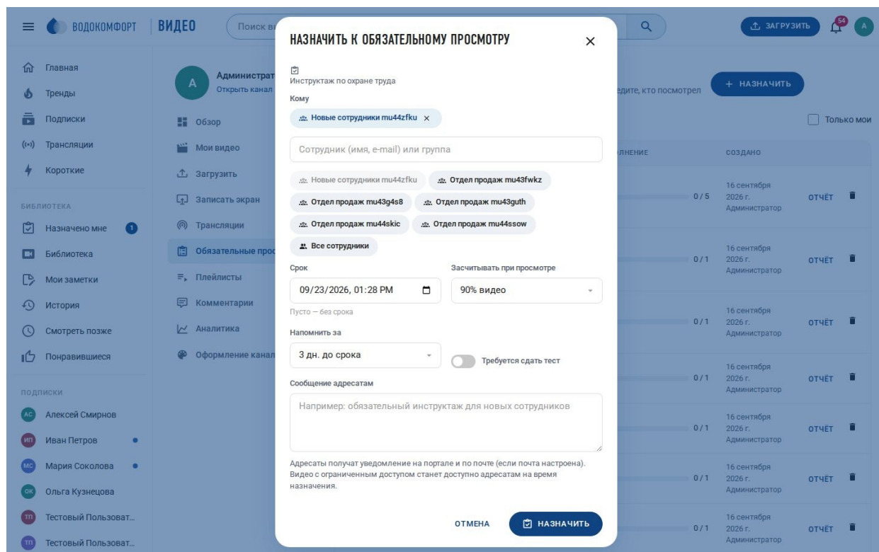
Рис. 44. Диалог назначения
