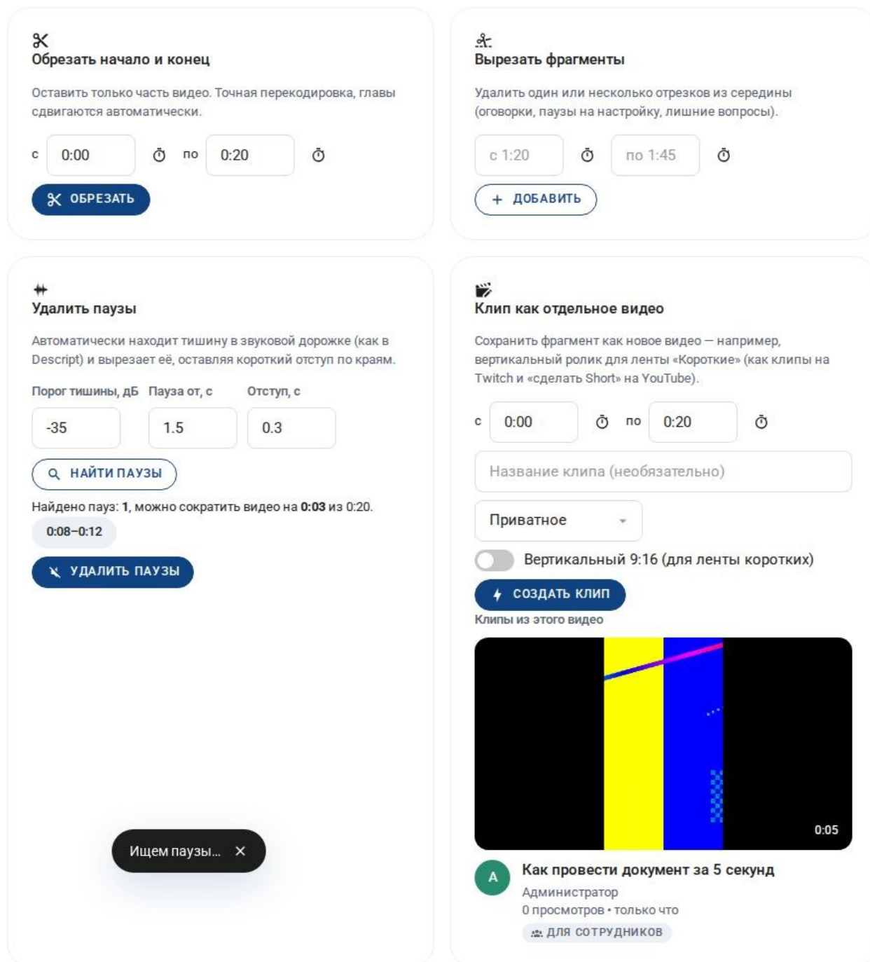
Рис. 76. Студия → Редактор
