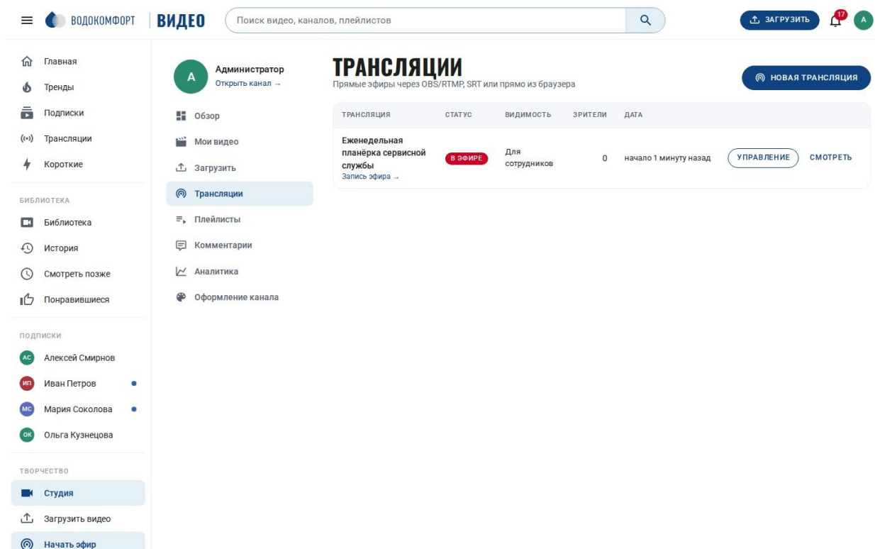
Рис. 37. Студия → Трансляции
