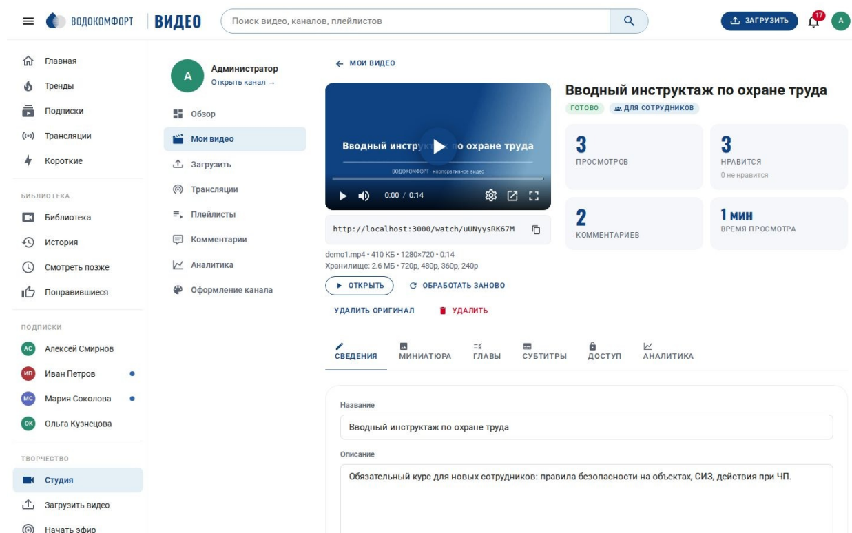
Рис. 34. Редактирование видео
